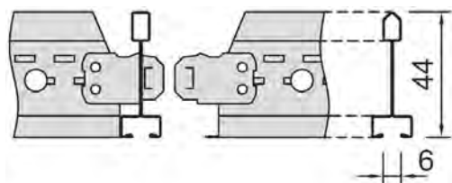
Silhouette XL 2 (Entrecalle 6 mm)
