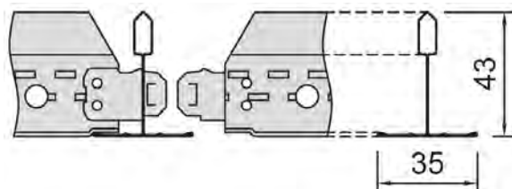
Silhouette XL 2 (Entrecalle 6 mm)
