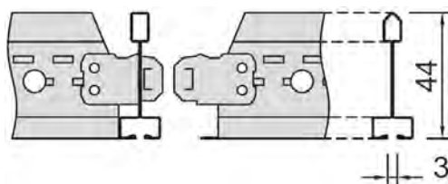
Silhouette XL 2 (Entrecalle 3 mm)
