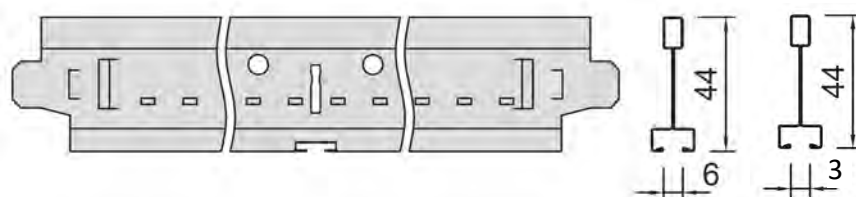
Primario Silhouette 15 mm Diseño entrecalle 6 mm y 3 mm
