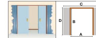
Puerta doble
