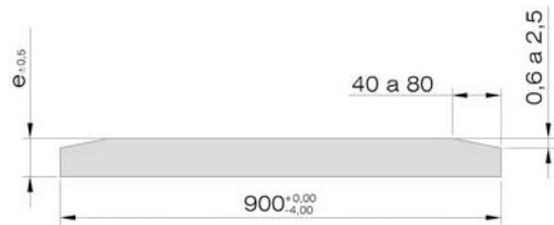
Cotas expresadas en mm.
